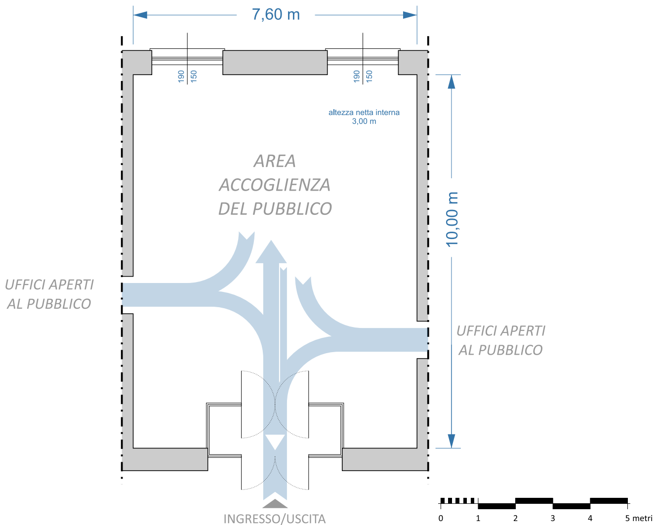
Schema planimetrico
